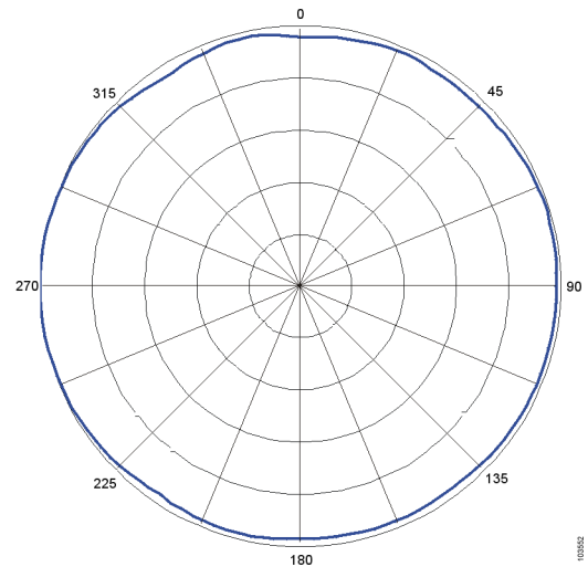
H-Plane Pattern
